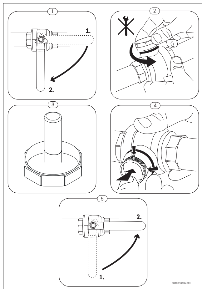
Bild 14 Siebreinigung
