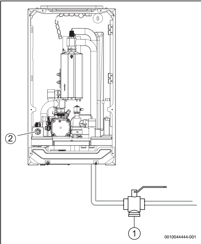
Bild 13 Inneneinheit Logatherm WLW176i/186i E
