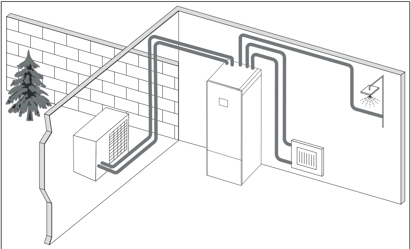
Bild 7 Wärmepumpe Logatherm WLW MB AR, Inneneinheit Logatherm WLW176i/186i T mit integriertem Warmwasserspeicher und elektrischem Zuluheizer
