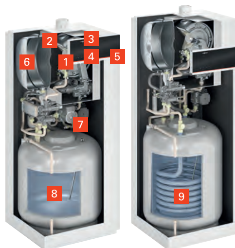
VITODENS 222-F (Typ B2TF)
